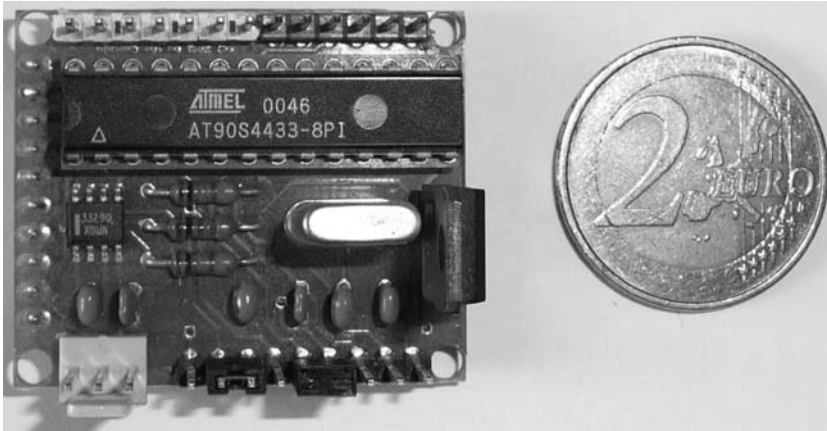
FIGURE 14.3 TTP/A node.
