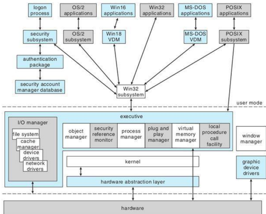
Gambar 4.3 Manajemen Proses
