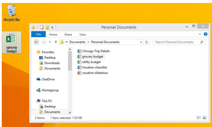
Gambar 13.45 Pencarian berkas
