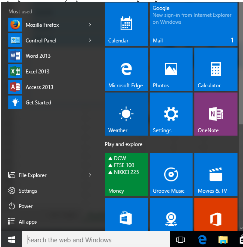
Gambar 13.64 Menu
