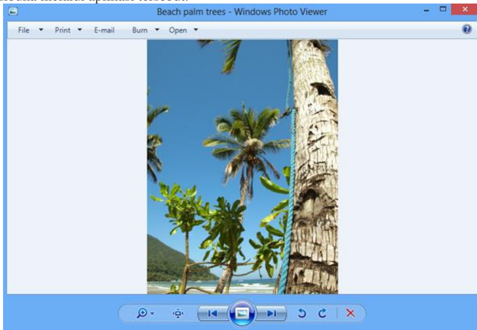
Gambar 13.70 Aplikasi Multimedia
