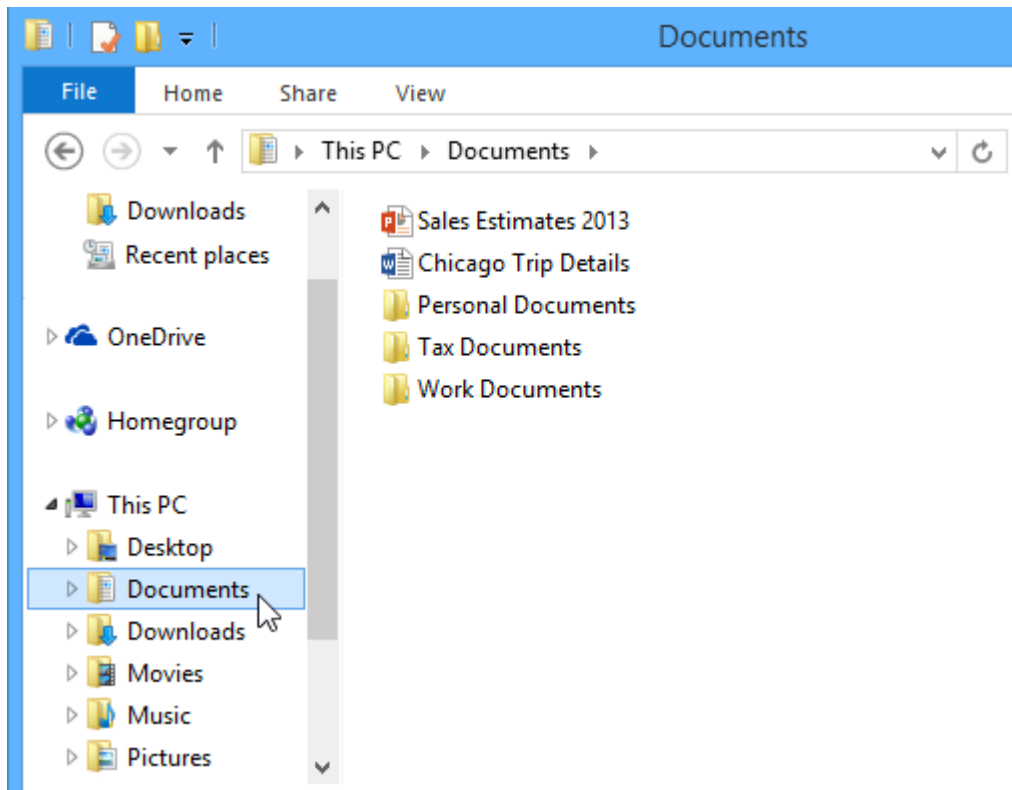
Gambar 13.37 Pencarian berkas
