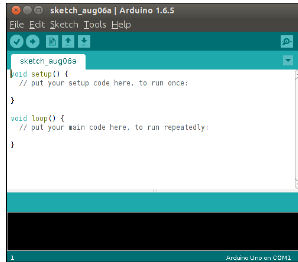
Figure 3 : Arduino IDE
