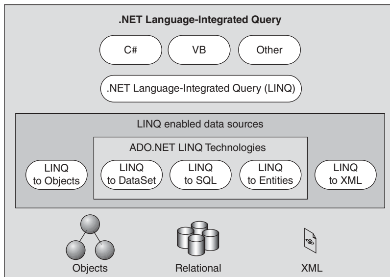
Figure 3.1. ADO.NET LINQ techniques.
